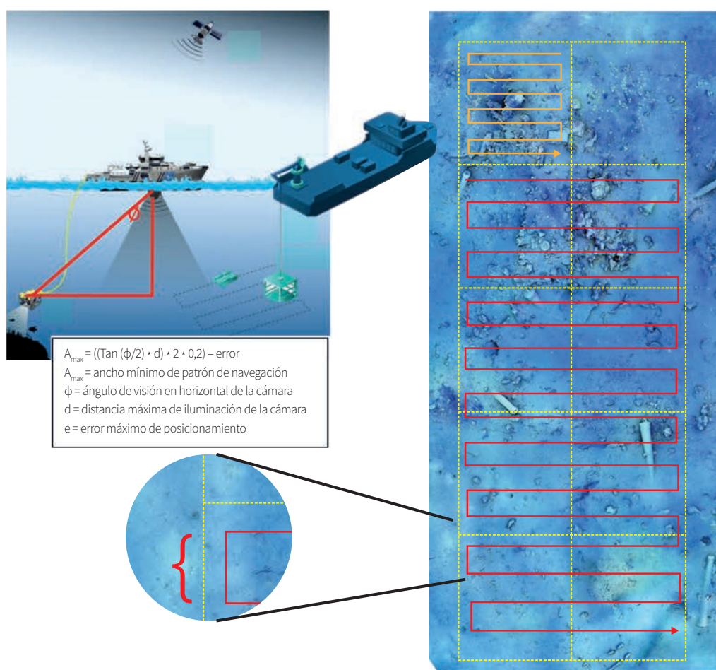
Figura 6. Cálculo de anchos del patrón de navegación y la velocidad máxima de navegación del roV
