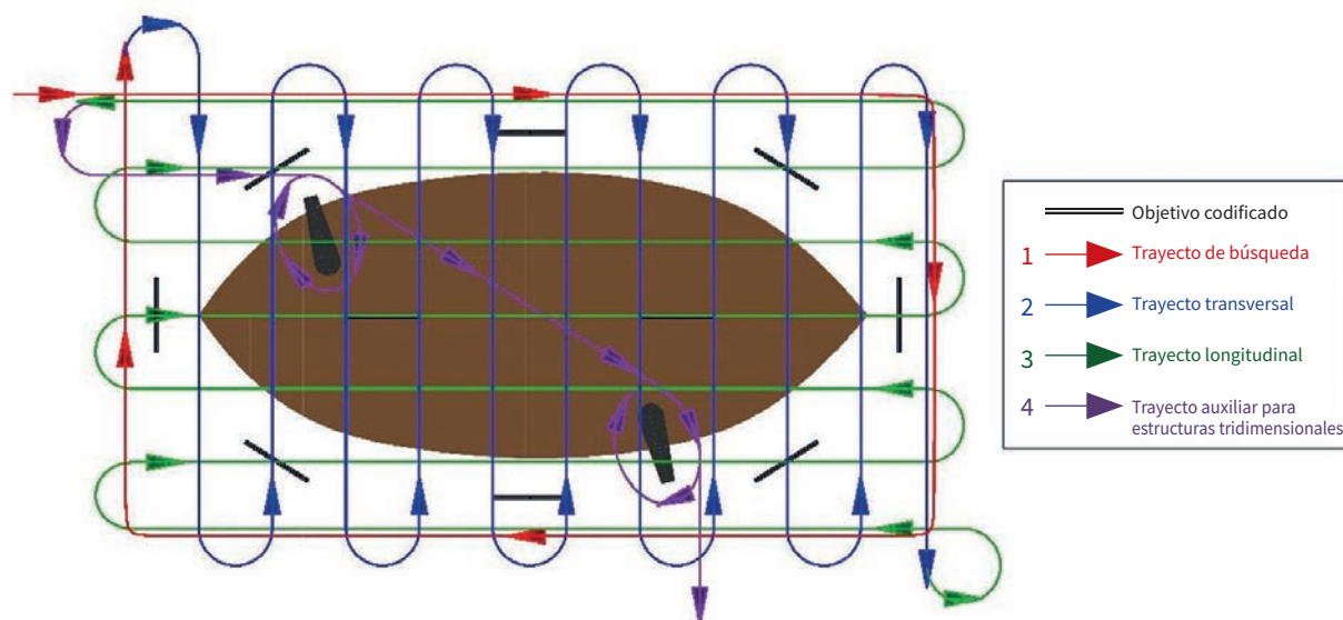
Figura 4. Modelo de patrón de navegación subacuático para el desarrollo de la fotogrametría
