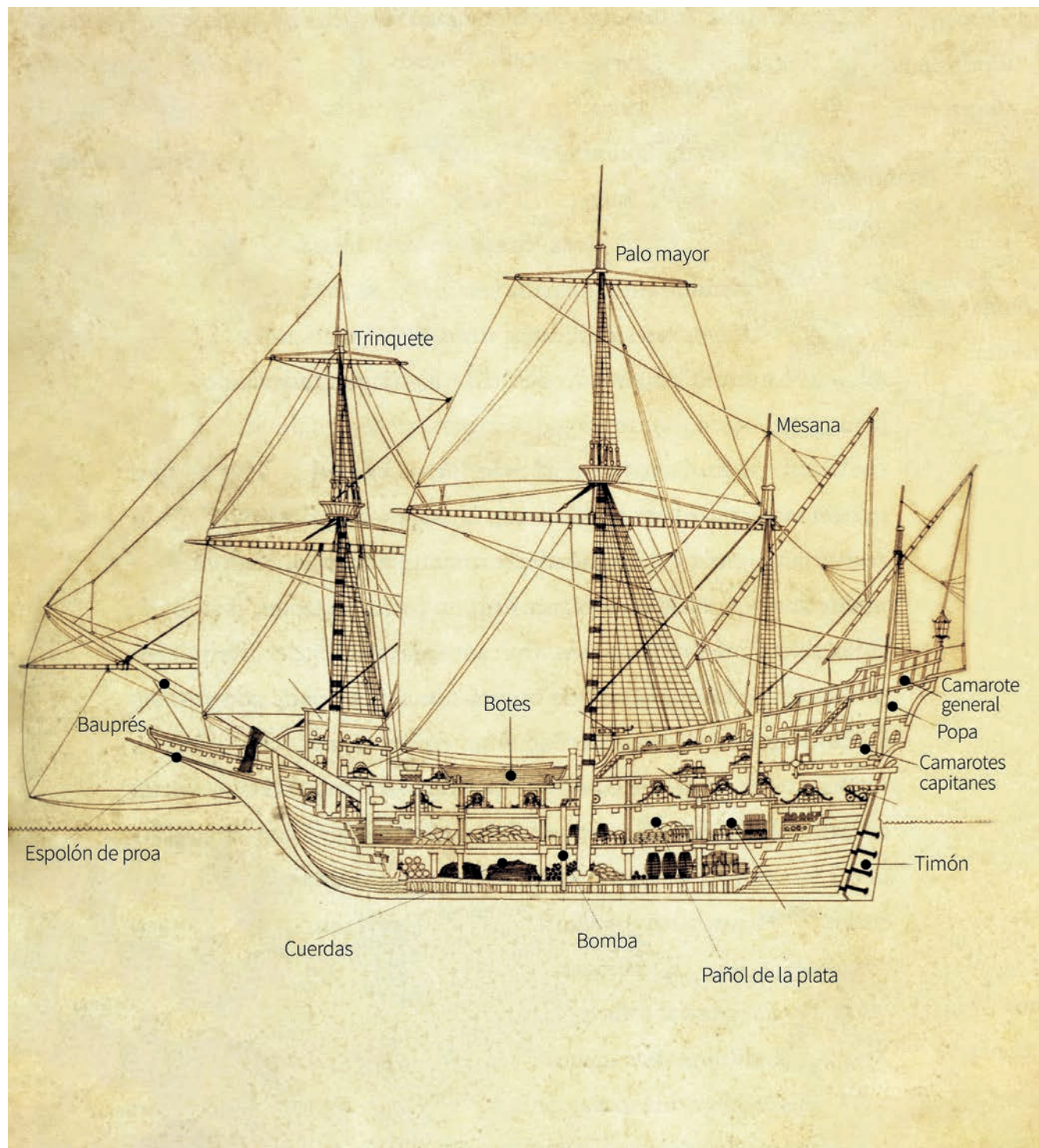
Figura 18. Esquema de las partes de un galeón
