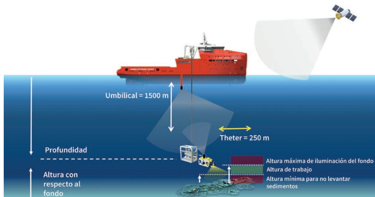
Figura 5. Proyección de campo de adquisición de datos
