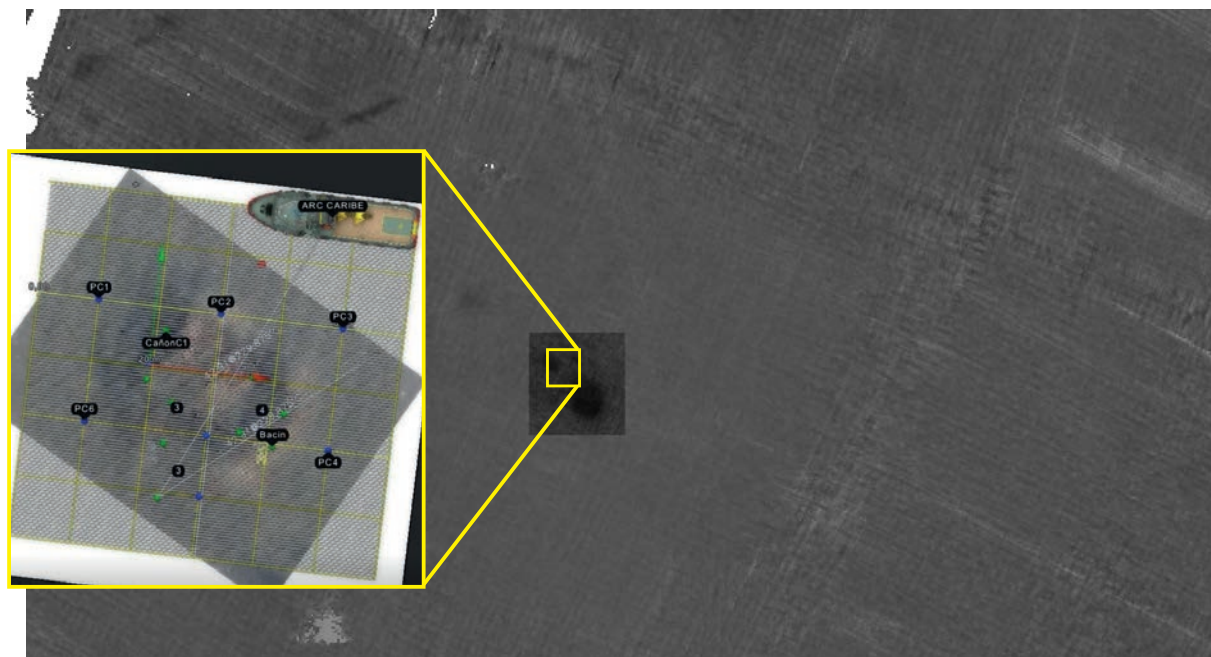
Figura 26. Mosaico Backscatter de la campaña hidrográfica de 2021
