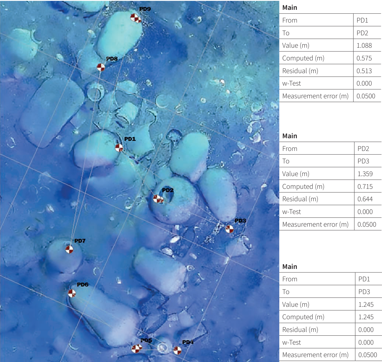
Figura 11. Mediciones realizadas en el contexto cultural a partir de los puntos de detalle en la popa del naufragio
