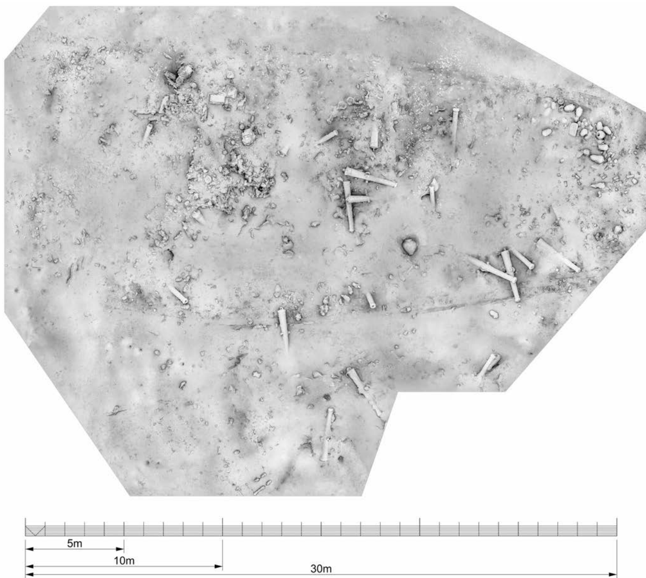
Figura 13. Modelo digital de elevación y modelo de escala de grises obtenidos a partir de procesamiento fotogramétrico
