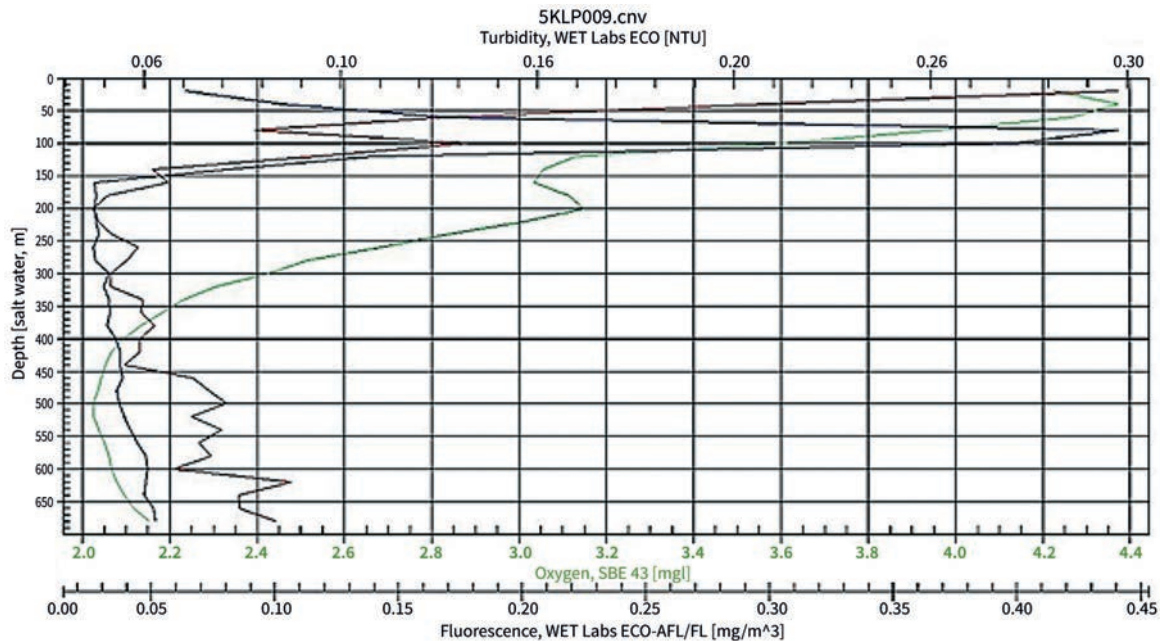
Figura 24. Perfil vertical de oxígeno disuelto (mg/l), turbidez (NTU) y fluorescencia de clorofila (mg/m 3 ) registrados en la estación 5KLP009
